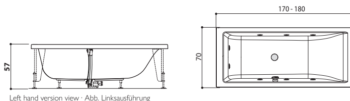
Left hand version view · Abb. Linksausführung
