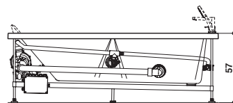
Left hand version view Abb. Linksausführung
