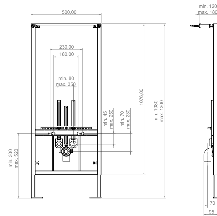
Монтажная рама для установки подвесного биде
