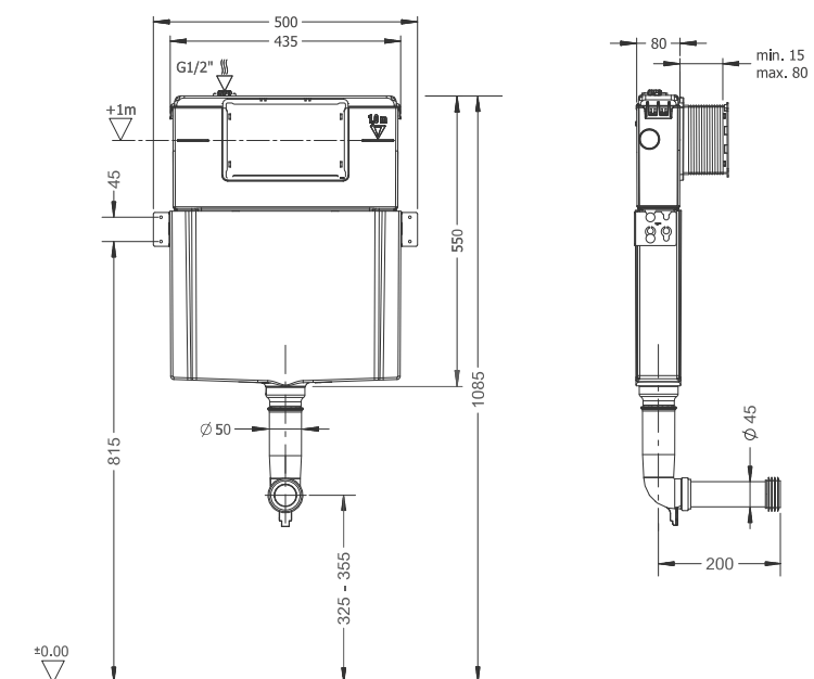
Смывной бак для напольного унитаза
