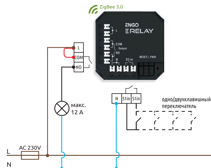
б) схема подключения для управления светом
