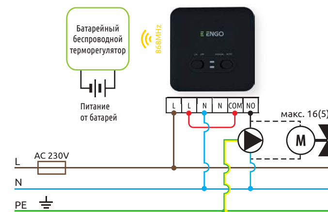
б) Схема подключения приёмника к насосу/сервоприводу
