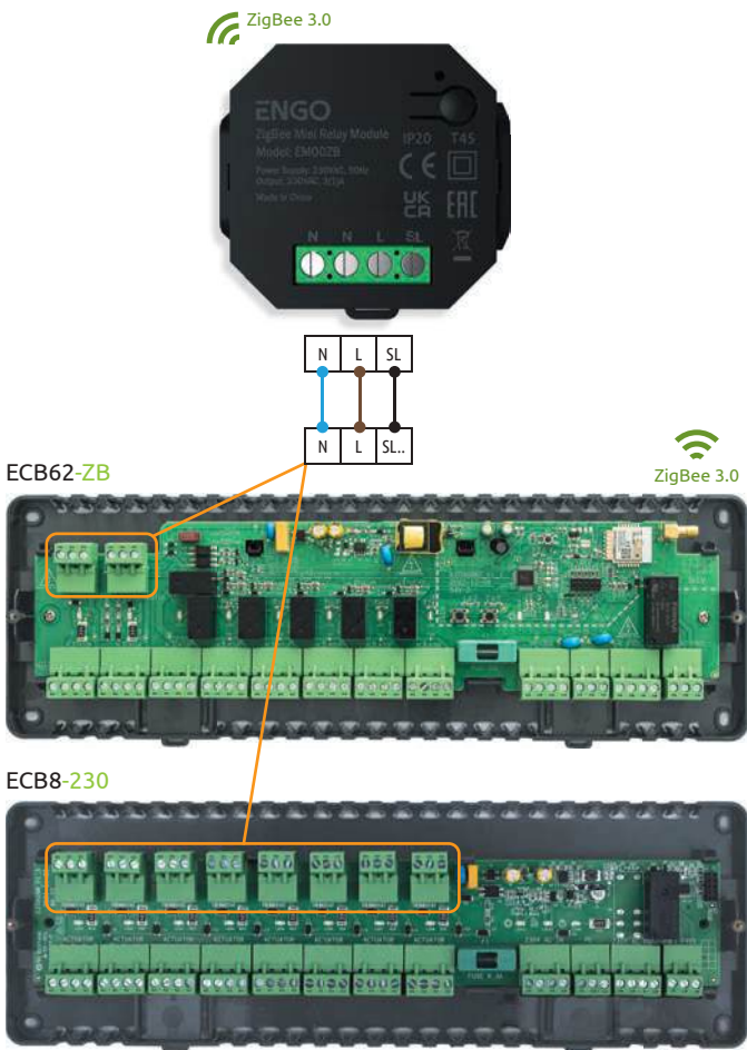
в) схема подключения к центру коммутации
