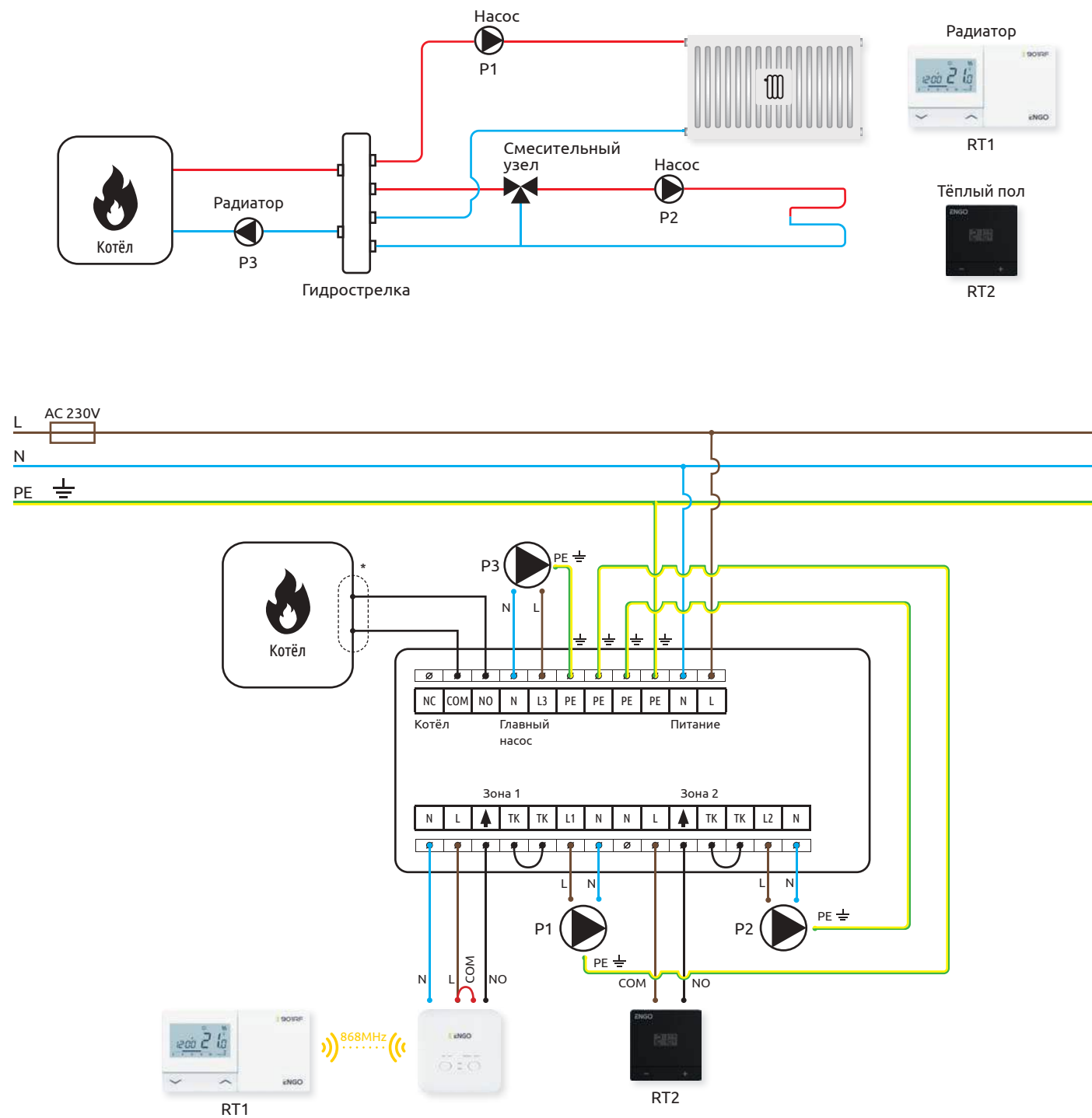
а) подключение двух контуров к центру коммутации
