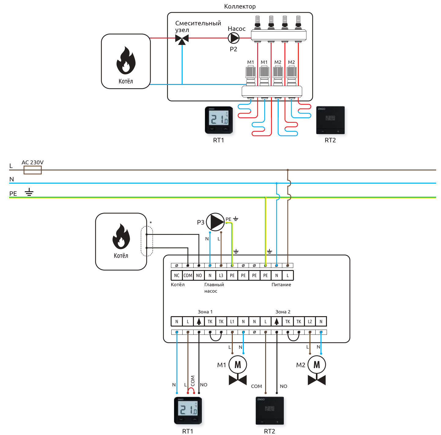
б) подключение двух зон тёплого пола к центру коммутации
