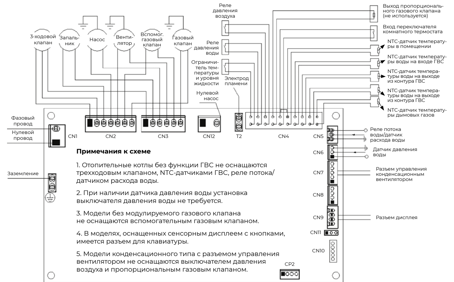
Рис. 26. Электрическая схема.
